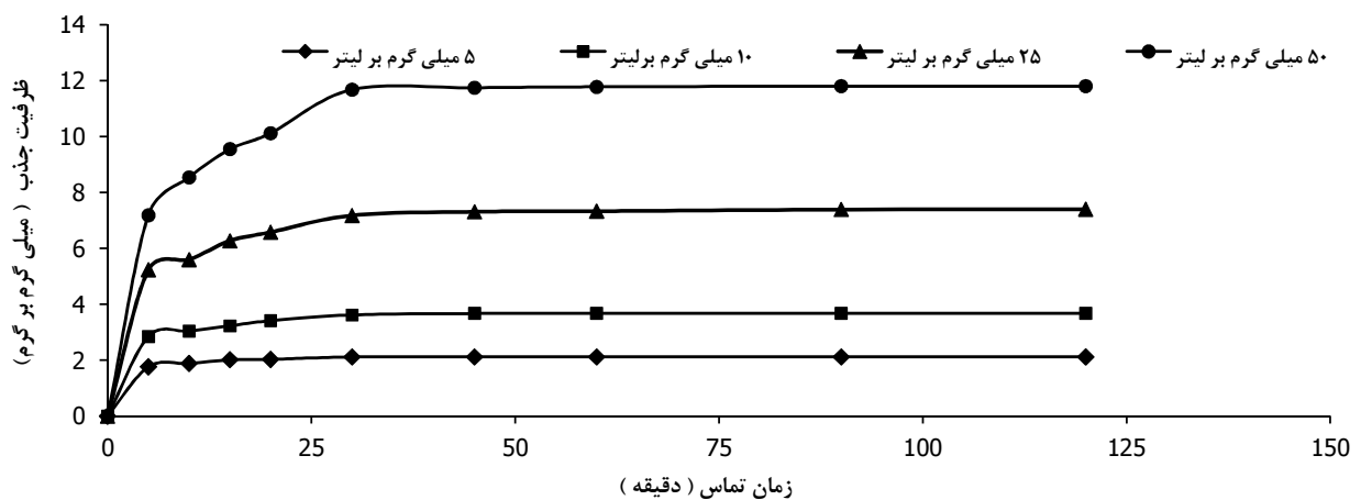
نمودار ۱: تأثیر زمان تماس و غلظت اولیه فنل بر میزان جذب فنل توسط MWCNTs ( pH = 5, M = 2\text{g/L}, C_0 = 5, 10, 25, 50\text{ mg/L} )
